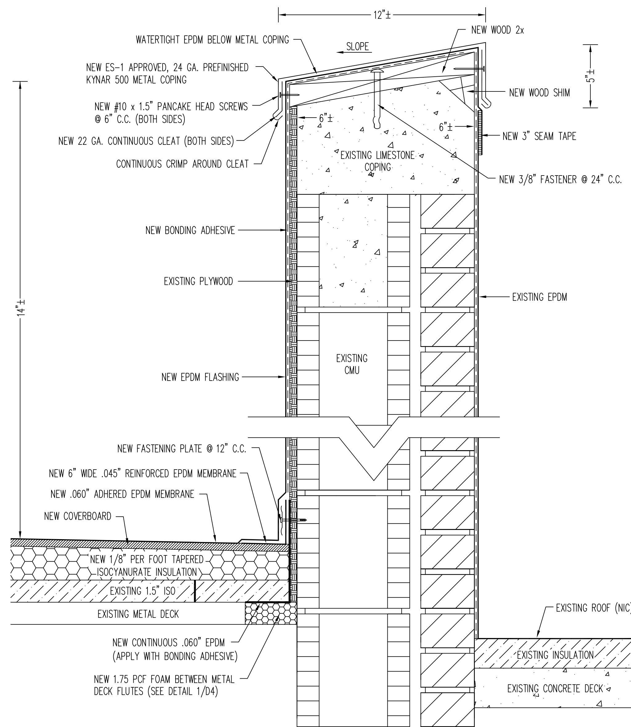
3 WALL FLASHING (PW) SCALE: 3" = 1'-0"
