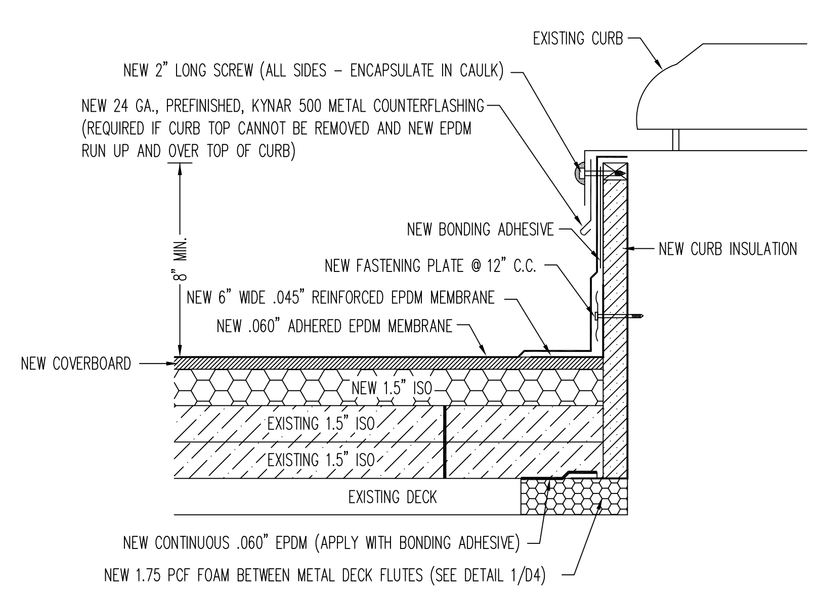
4 CURB DETAIL SCALE: 3" = 1'-0"
