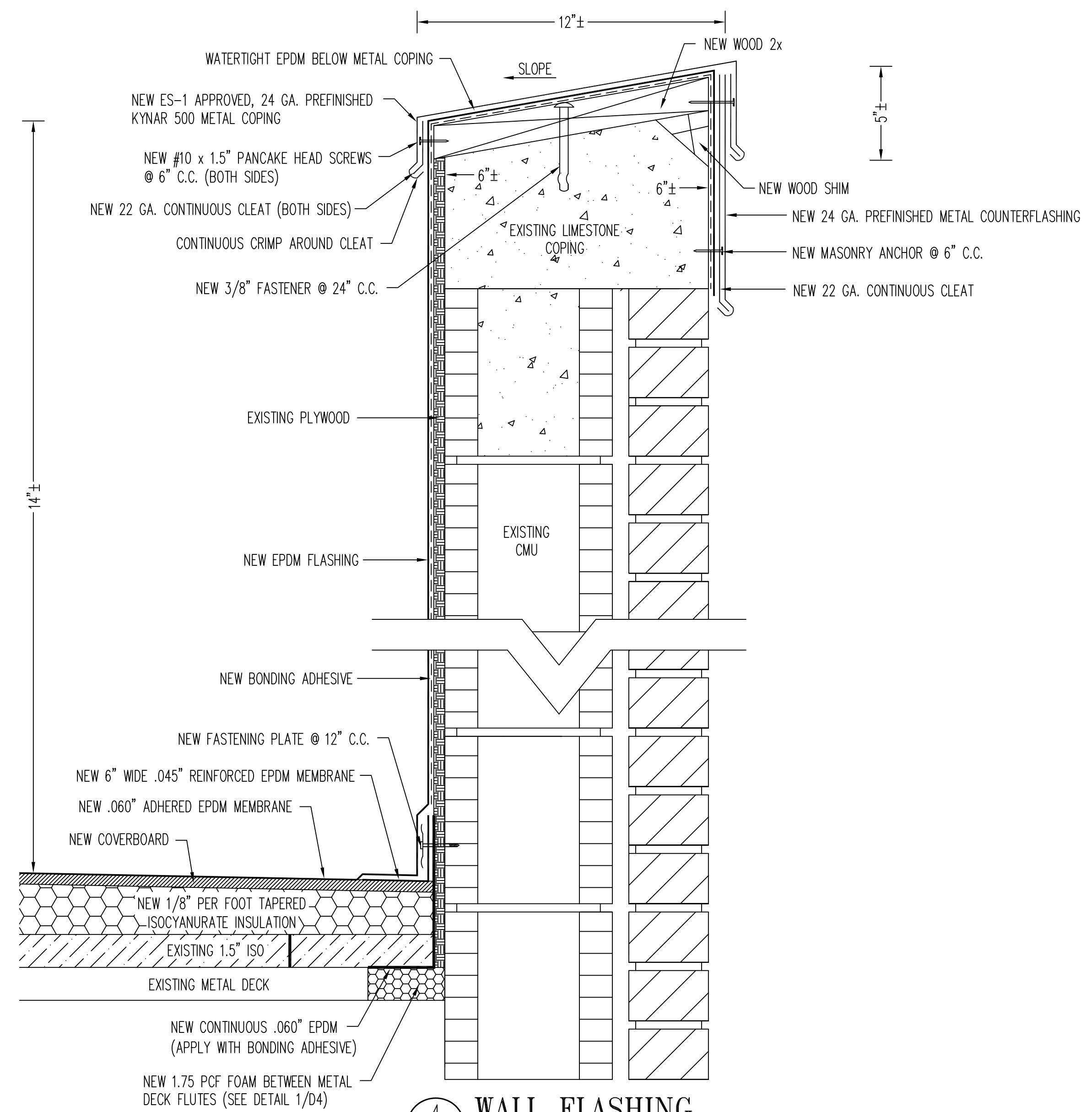
4 WALL FLASHING (PW) SCALE: 3" = 1'-0"
