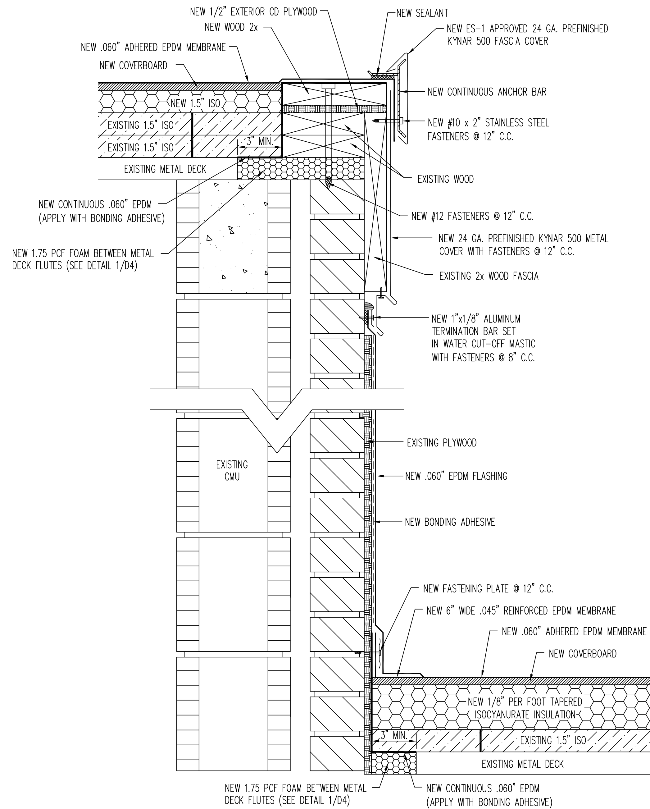
1 WALL FLASHING SCALE: 3" = 1'-0"
