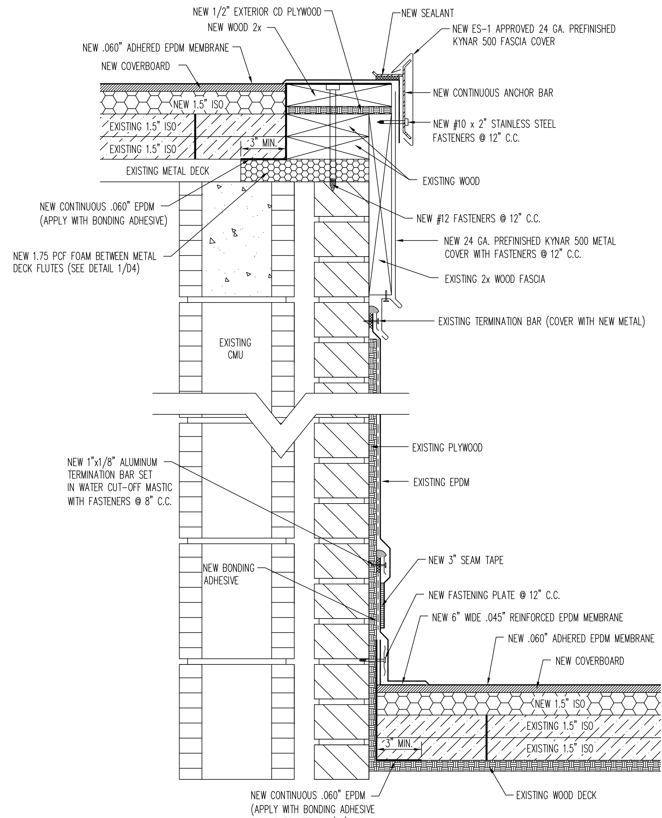
2 WALL FLASHING SCALE: 3" = 1'-0"
